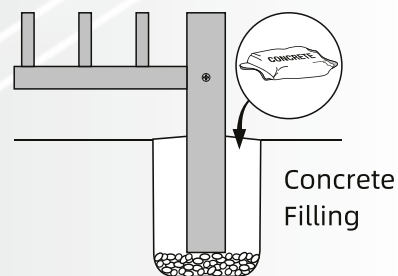
3 Set Post 安装立柱, 注入水泥
