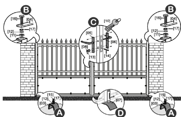
安装示意图 Instal Indicating
