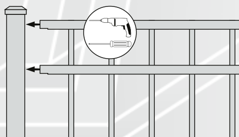
2 Install Panel 安装栅栏
